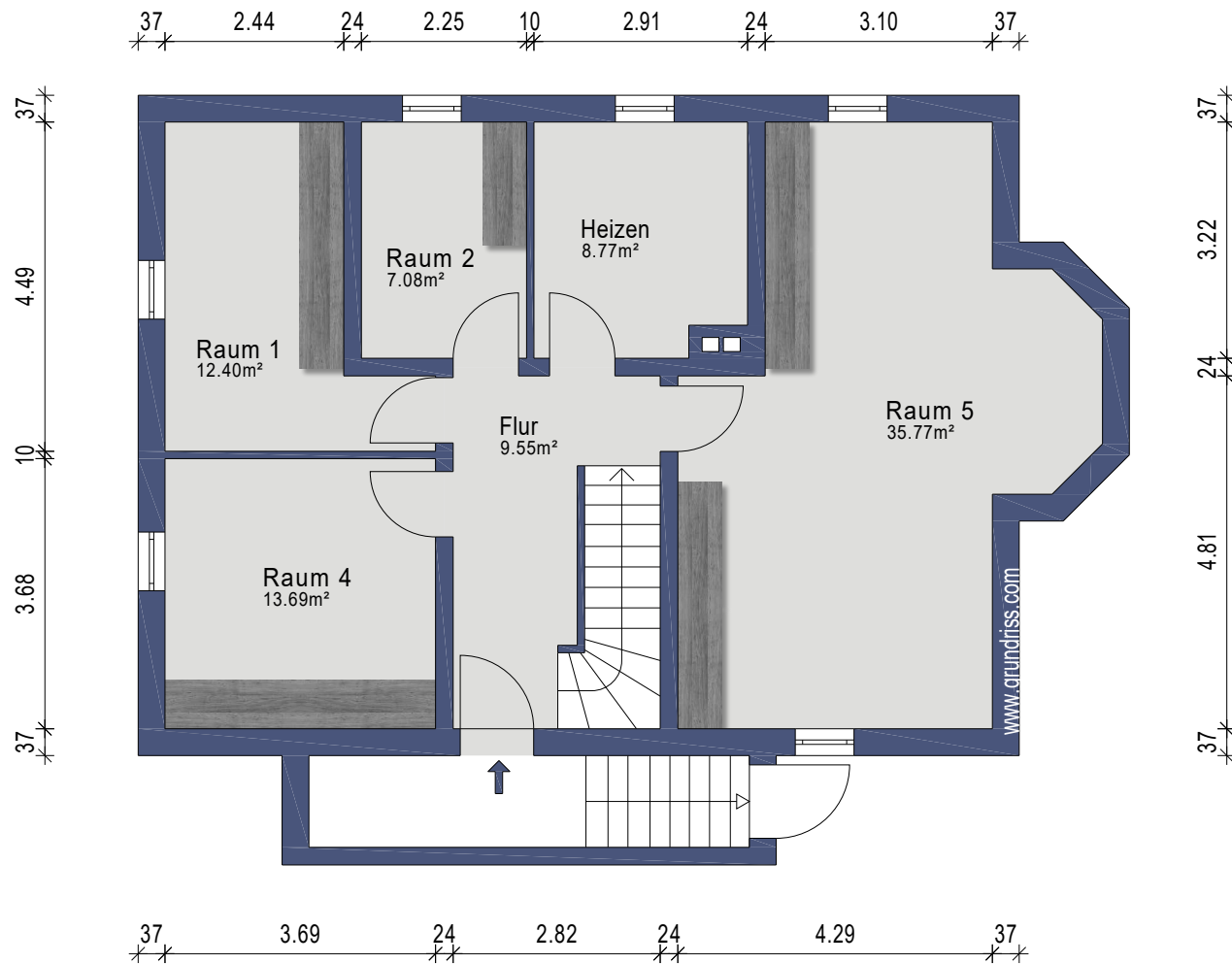
Kellergeschoss
